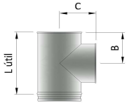
BITW TE 90° CON INJERTO HEMBRA TEE 90° FEMALE CONNECTION
