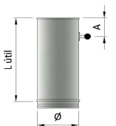
BIDA COMPUERTA 0,5 m CON TIRADOR HANDLE DAMPER 0,5 m
