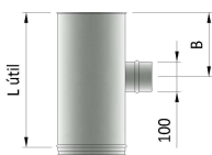
BITJ TE DE 0,5 m REGISTRO Ø100 Ø100 INSPECTION TEE 0,5 m
