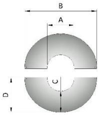
HIPU PLACA EMBELLECEDORA REDONDA 150 90° ROUND FINISHING PLATE 150 90°
