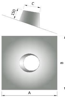
HICR CUBREAGUAS DE PLOMO 0°- 20° LEAD FLASHING 0°- 20°
